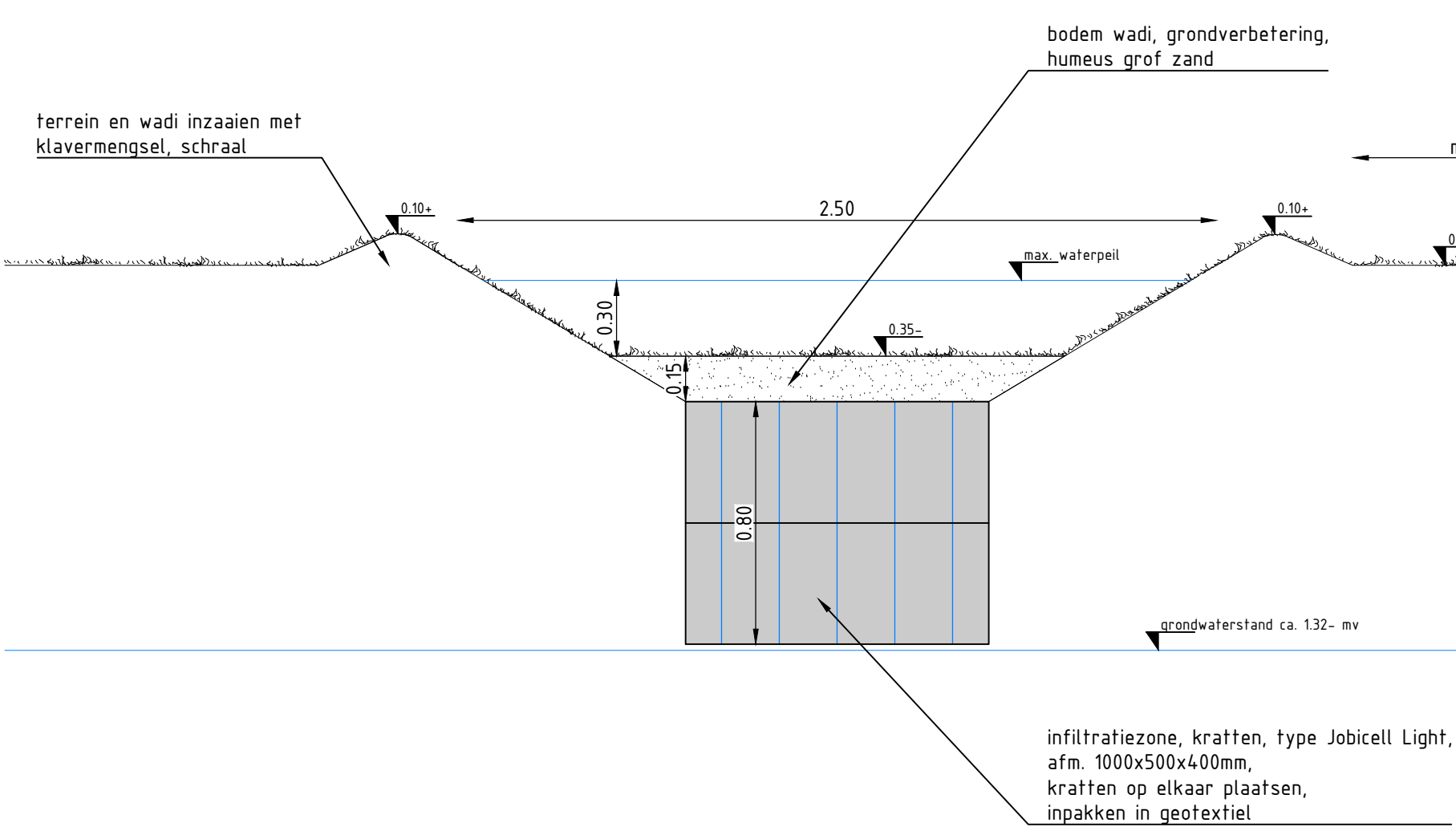
Principedoorsnede B-B' schaal 1:20
